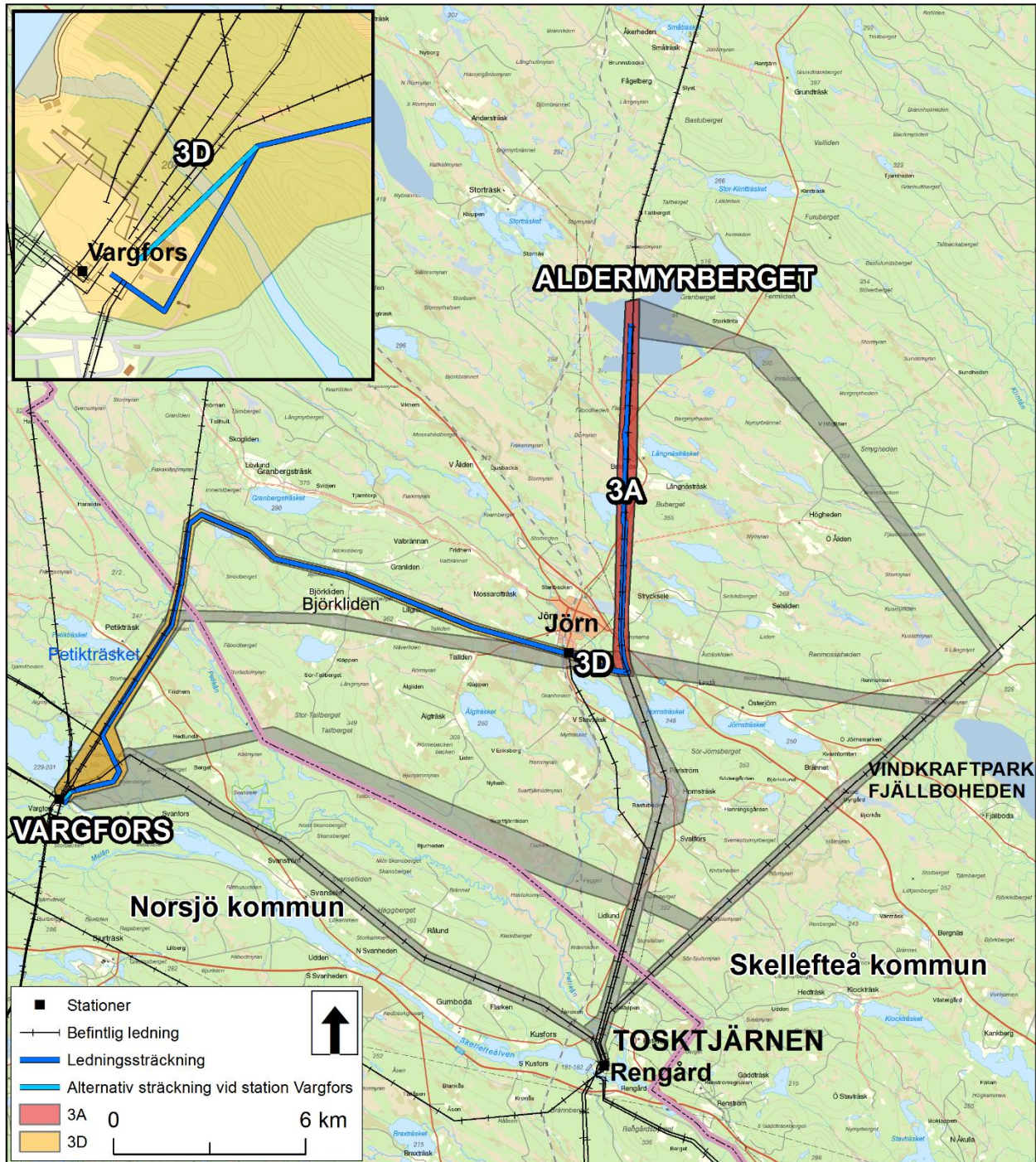
Figur 1. Karta över de stråk som Vattenfall Elddistribution väljer att gå vidare med och söka koncession för ny ledning inom, samt de stråk som utesluts från den fortsatta utredningen (grå stråk). Föreslagen ledningssträckning mellan Aldermyrberget och Vargfors markeras med blått streck.
