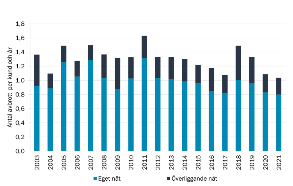
Figur 5 Genomsnittligt antal långa oaviserade avbrott per kund och år (SAIFI) för perioden 2003–2021
