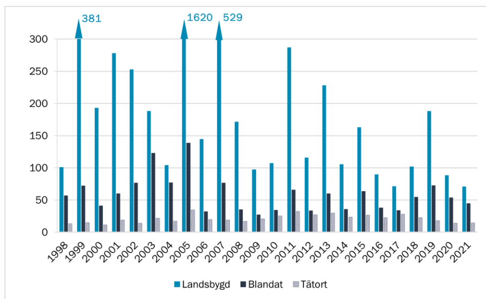
Figur 17 Genomsnittlig avbrottstid i minuter per år i det egna nätet fördelat på landsbygdsnät, blandat nät och tätortsnät (SAIDI) för perioden 1998–2021
