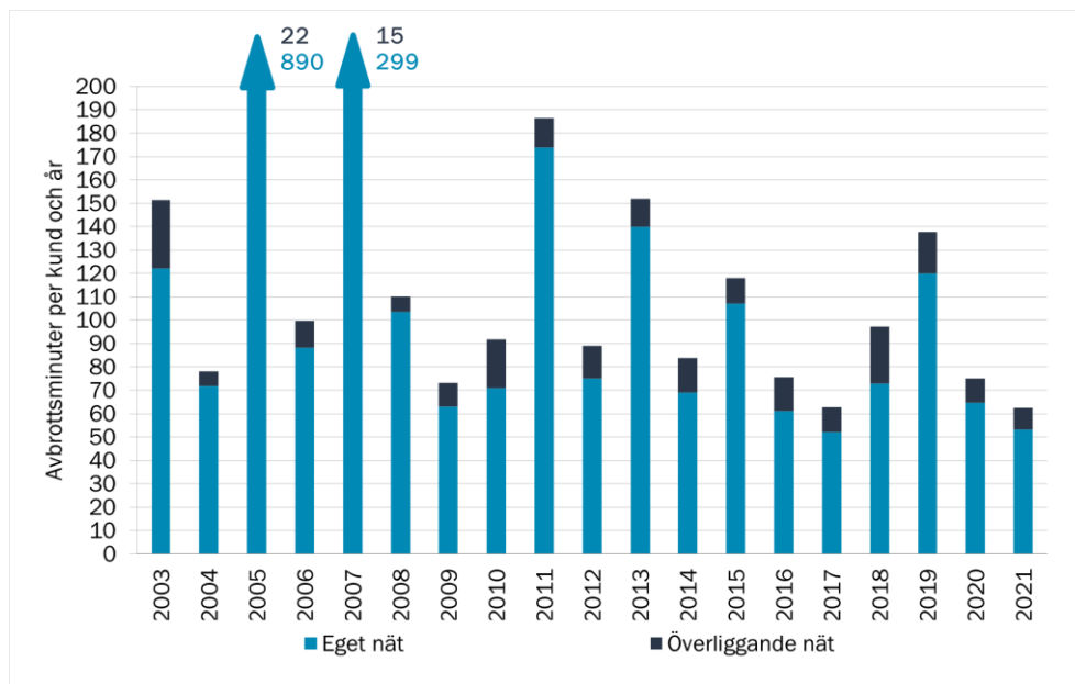
Figur 6 Genomsnittlig avbrottstid i minuter för långa oaviserade avbrott per kund och år (SAIDI) för perioden 2003–2021
