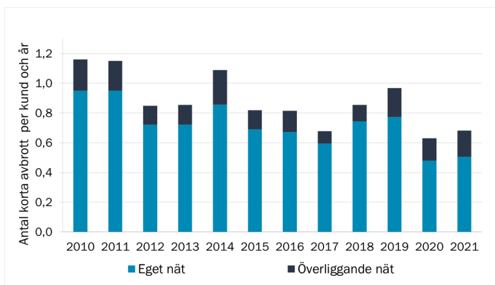
Figur 11 Genomsnittligt antal korta avbrott per kund och år (MAIFI) för perioden 2010–2021
