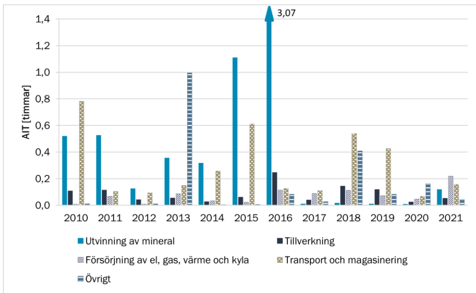
Figur 30 Avbrottstid avseende oaviserade avbrott >3 minuter (AIT) för olika kundkategorier (effektviktat medelvärde) för perioden 2010–2021
