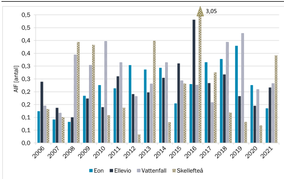
Figur 31 Effektivtade medelvärde av antal oaviserade långa avbrott per regionnätSFöretag (AIF) för perioden 2006–2021
