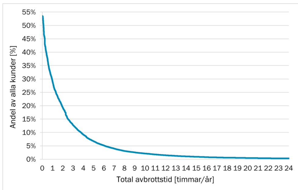
Figur 10 Andel kunder med en sammanlagd årlig avbrottsid om x timmar eller längre (CELID-t) 2021
