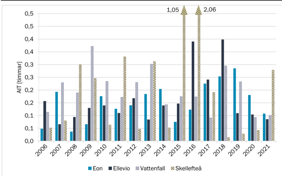
Figur 32 Avbrottsstid avseende oaviserade avbrott >3 minuter (AIT) per regionnätstföretag (effektviktat medelvärde) för perioden 2006–2021
