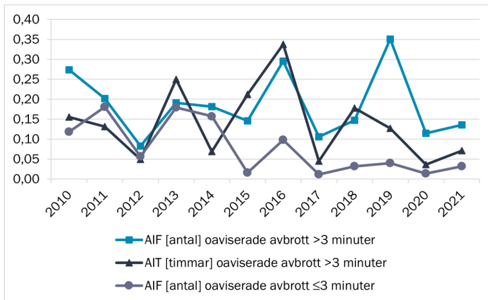
Figur 28 Avbrottsindikatorer för kunder anslutna direkt till regionnät för perioden 2010–2021
