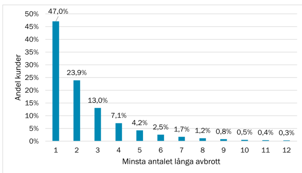
Figur 7 Andel kunder med x antal avbrott eller fler (CEMI-X) 2021
