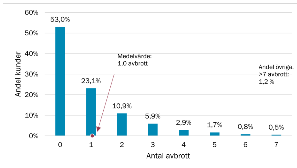
Figur 4 Fördelning av antal långa oaviserade avbrott för enskilda kunder 2021. Medelvärdet markeras med en röd punkt
