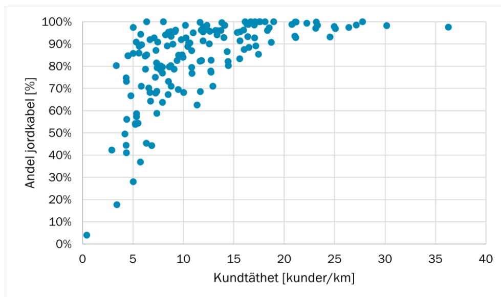
Figur 18 Illustration av sambandet mellan andelen jordkabel och respektive elnäts kundtätthet 2021
