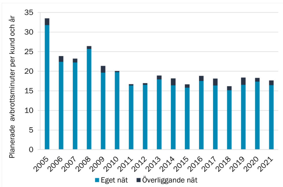
Figur 22 Avbrottstid i minuter per kund och år (SAIDI) för aviserade avbrott för perioden 2005–2021
