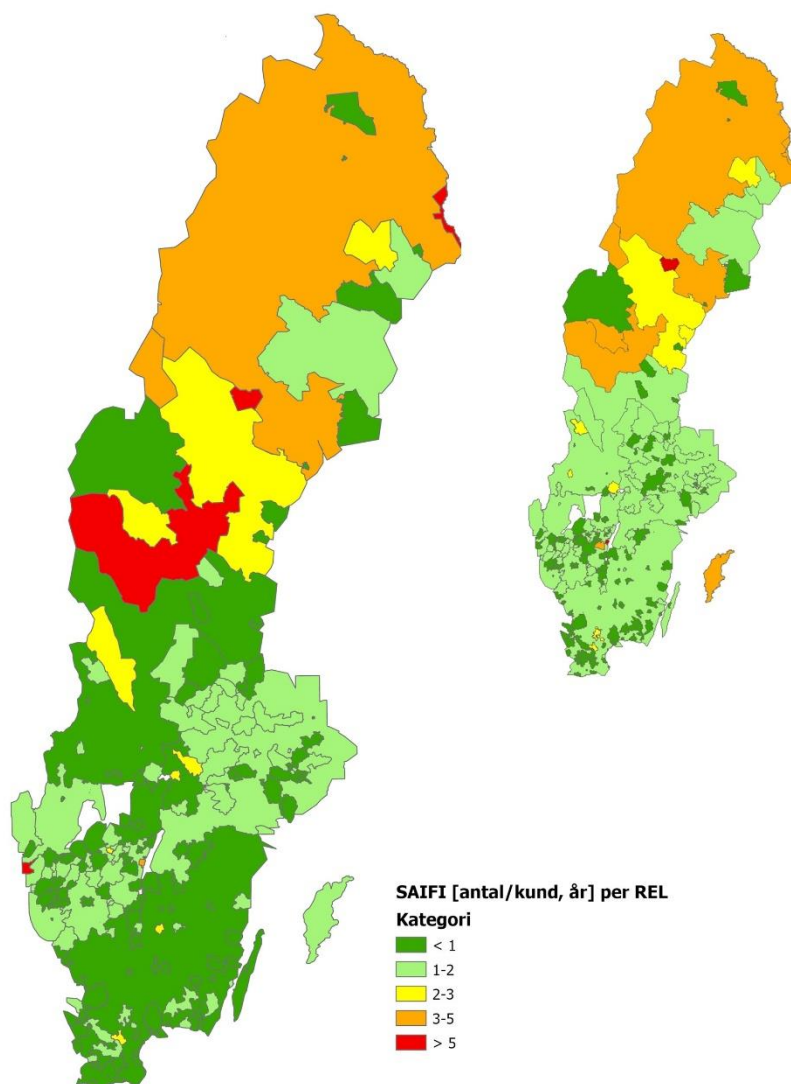
Figur 23 Genomsnittligt antal avbrott >3 min per kund (SAIFI) per redovisningsenhet 2021 (miniatyrkarta för jämförelse med 2020)
