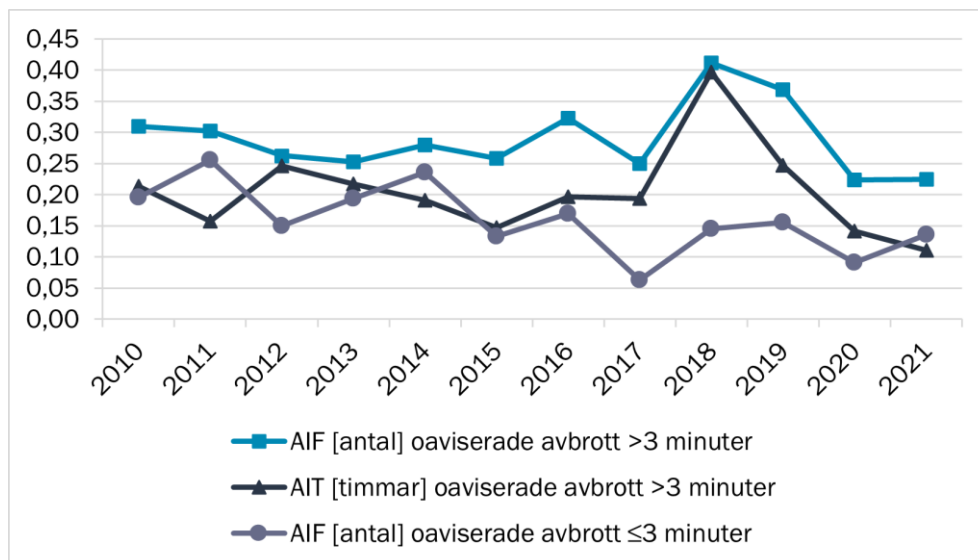
Figur 27 Avbrottsindikatorer för regionnätens gränspunkter avseende oaviserade avbrott för perioden 2010–2021
