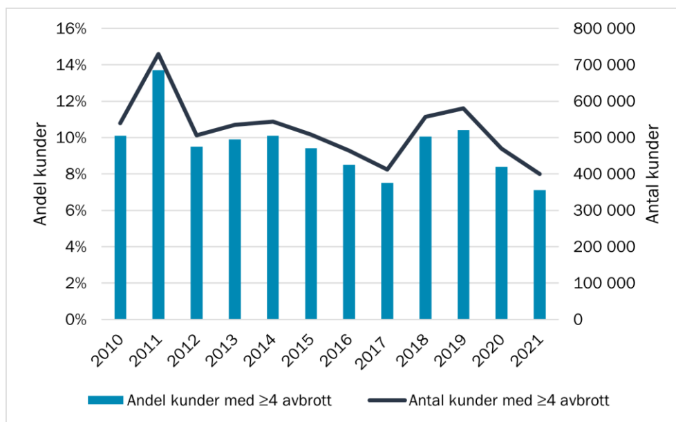
Figur 8 Andelen och antalet kunder med fyra eller fler avbrott per år (CEMI-4) för perioden 2010–2021
