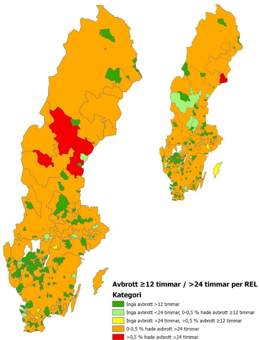
Figur 25 Avbrott längre än 12 respektive 24 timmar under 2021 (miniatyrkarta för jämförelse med 2020) per redovisningsenhet
