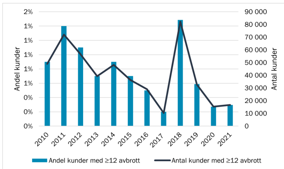
Figur 9 Andelen och antalet kunder med tolv eller fler avbrott per år (CEMI-12) för perioden 2010–2021
