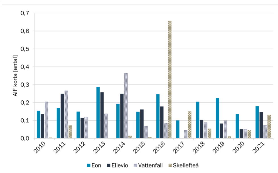
Figur 33 Effektviktade medelvärden avseende antal korta avbrott per företag och år (AIF avseende ≤3 min) för perioden 2010–2021
