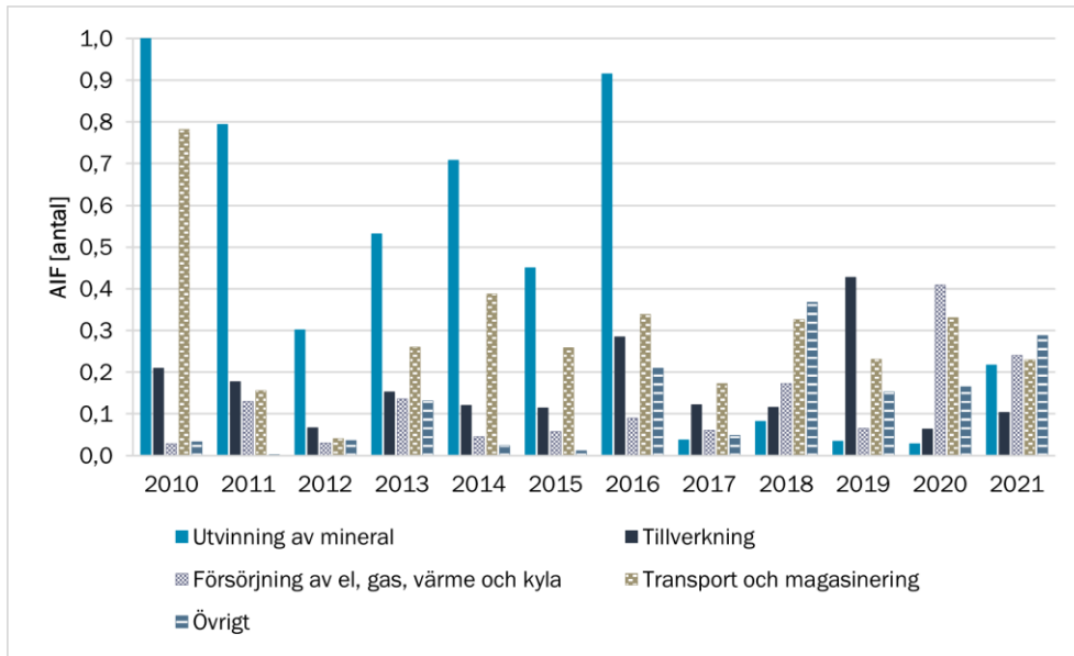
Figur 29 Antal oaviserade avbrott >3 minuter (AIF) för olika kundkategorier (effektviktat medelvärde) för perioden 2010–2021
