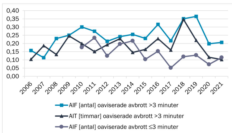
Figur 26 Avbrottsindikatorer för regionnätets samtliga anläggningspunkter avseende oaviserade avbrott för perioden 2006–2021
