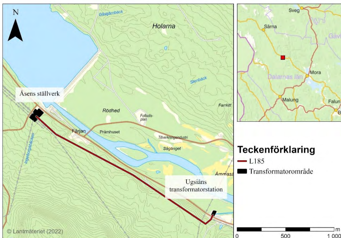
Figur 1. Befintlig 72,5 kV luftledning L185. Ledningen går mellan Åsens ställverk och Ugsiåns transformatorstation.
