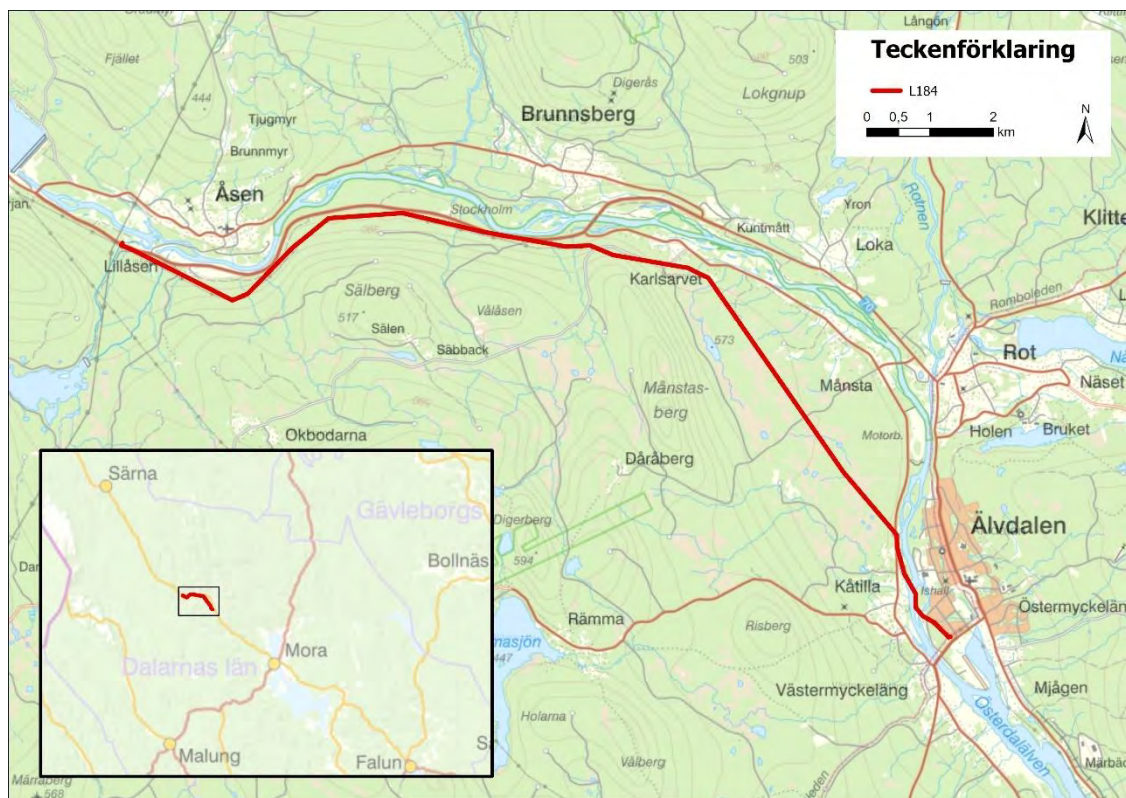
Figur 1. Befintlig 72,5 kV luftledning, L184, mellan Ugsiås transformatorstation och Älvdalens transformatorstation.
